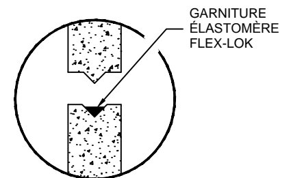
DÉTAIL DU JOINT
