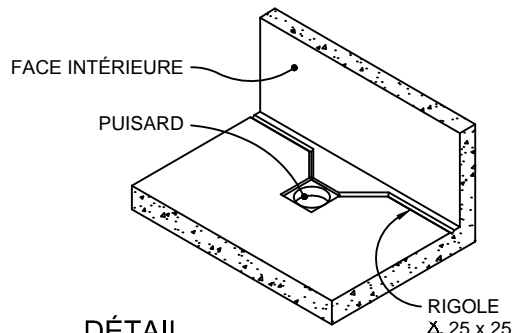
DÉTAIL DU PUISARD & RIGOLE
