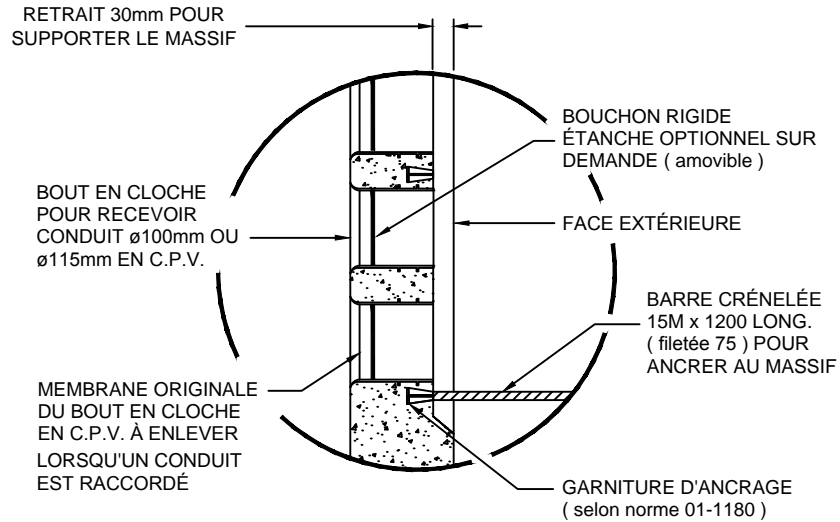
DÉTAIL DU BOUT EN CLOCHE
