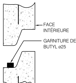
DÉTAIL 8
