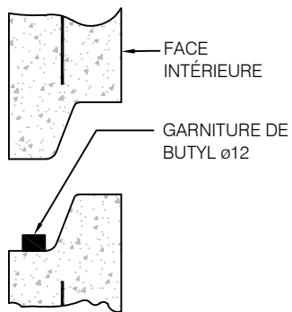
DÉTAIL 4
