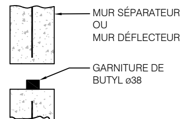
DÉTAIL 10
