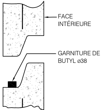
DÉTAIL 1
