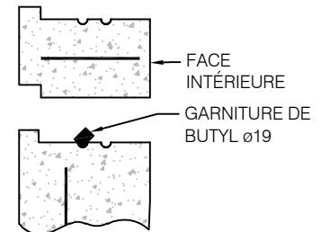
DÉTAIL 6
