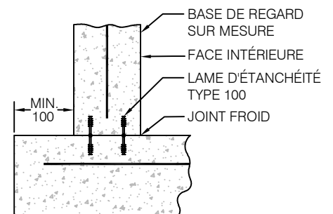
DÉTAIL 9
