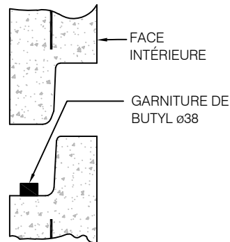
DÉTAIL 5
