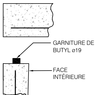
DÉTAIL 7
