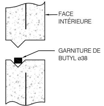
DÉTAIL 3
