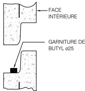
DÉTAIL 2
