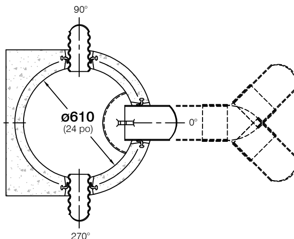
BASE DU PUISARD (ANGLES DISPONIBLES)
