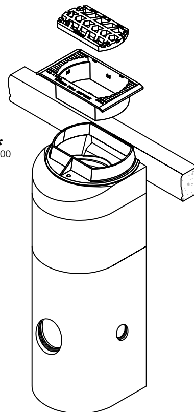
VUE EN ISOMÉTRIE
