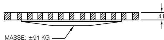
GRILLE ANTI-VÉLO
