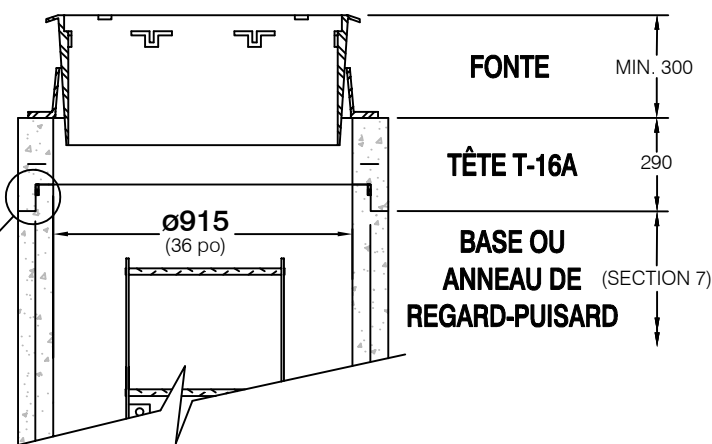
GRILLE
