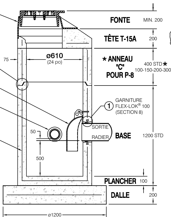
BASE DU PUISARD (ANGLES DISPONIBLES)
