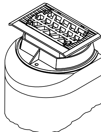
TÊTE "T-15A" POUR GRILLE RECTANGULAIRE 352 x 581 MM
