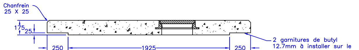
ÉLÉVATION
